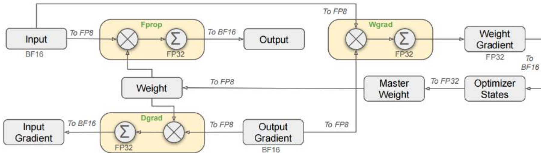
图：采用FP8数据格式的整体混合精度框架
