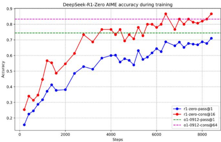
图：DeepSeek-R1-Zero训练中针对AIME正确率持续提高
