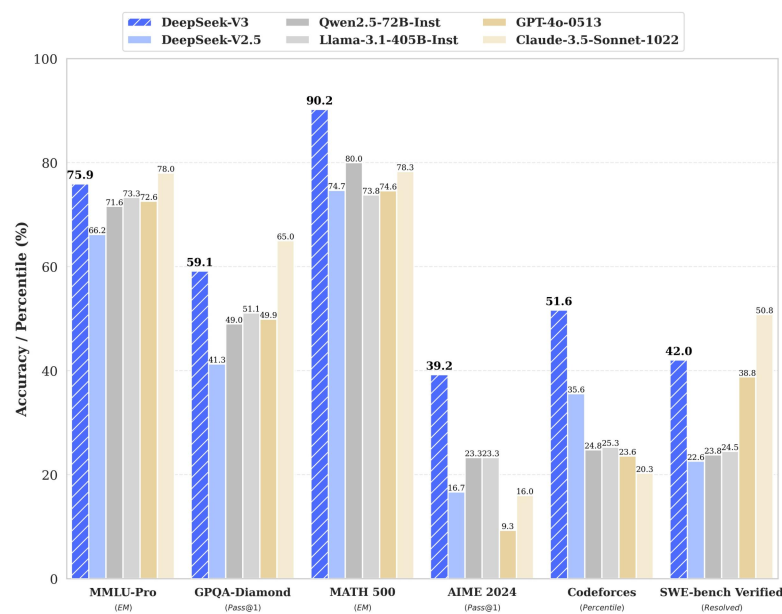
图：DeepSeek-V3等模型执行不同推理任务性能对比
