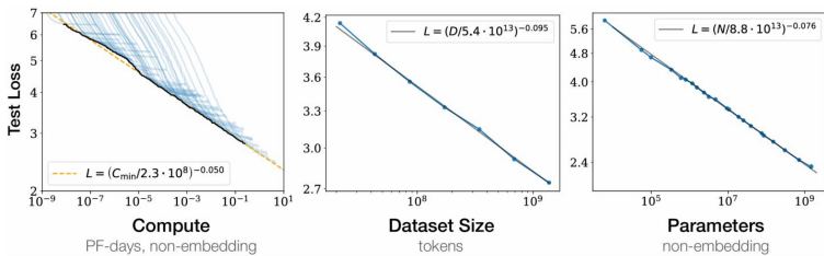
图：模型规模的指数提升线性提高模型性能
