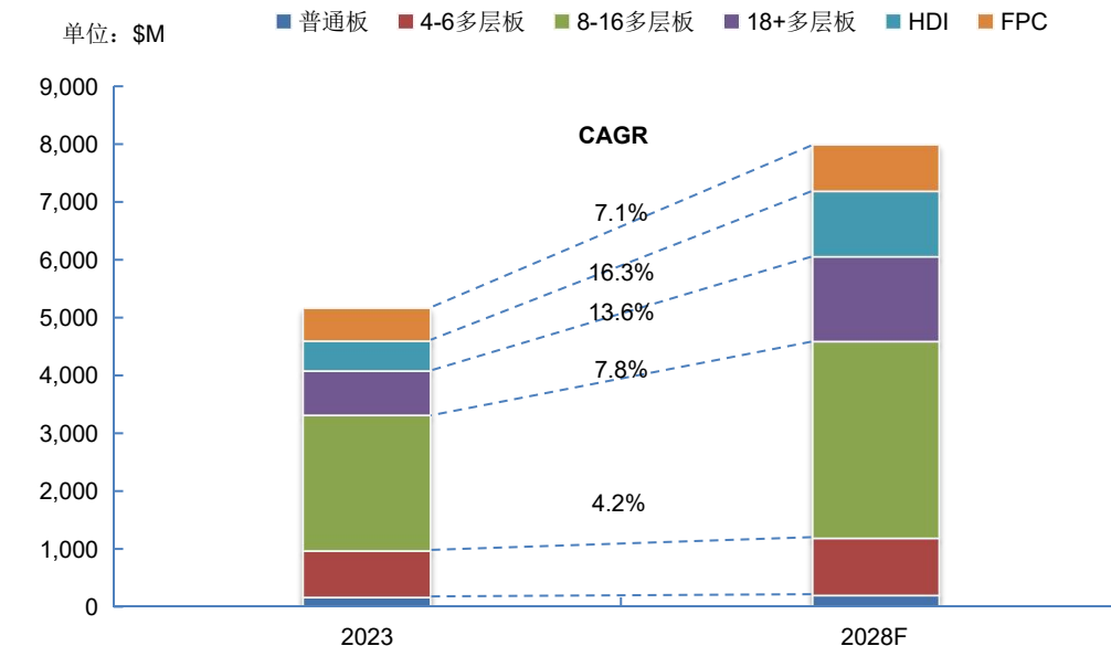
图：服务器PCB市场分产品占比
