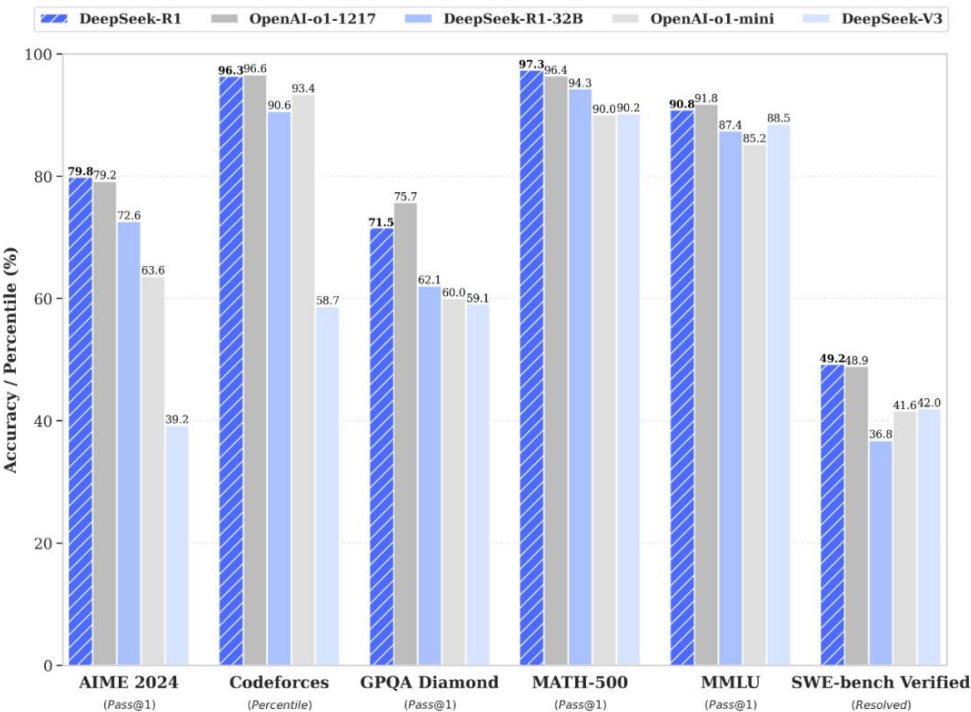
图：DeepSeek-R1等模型执行不同推理任务性能对比
