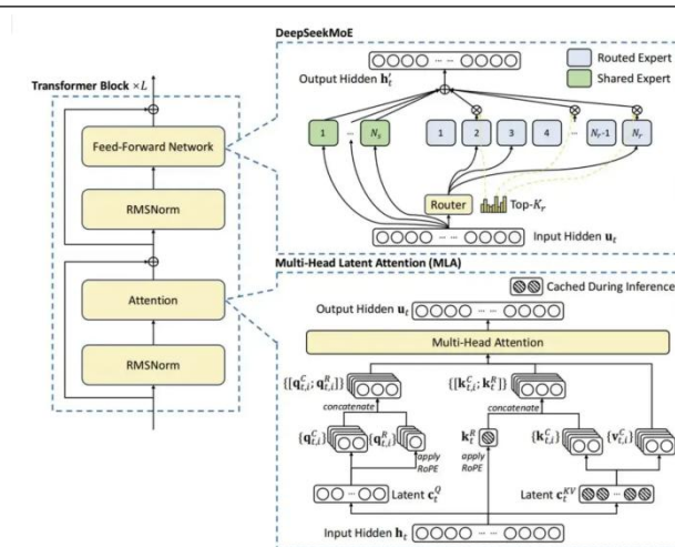
图2: Deepseek 的 MLA 和 MoE 架构
