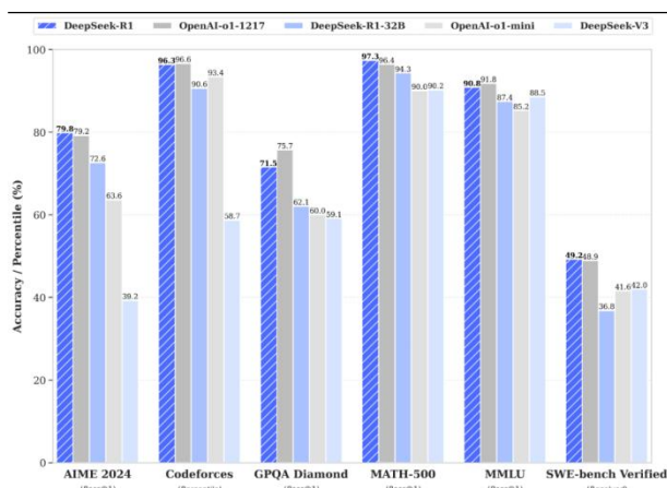
图7: Deepseek-R1 性能
